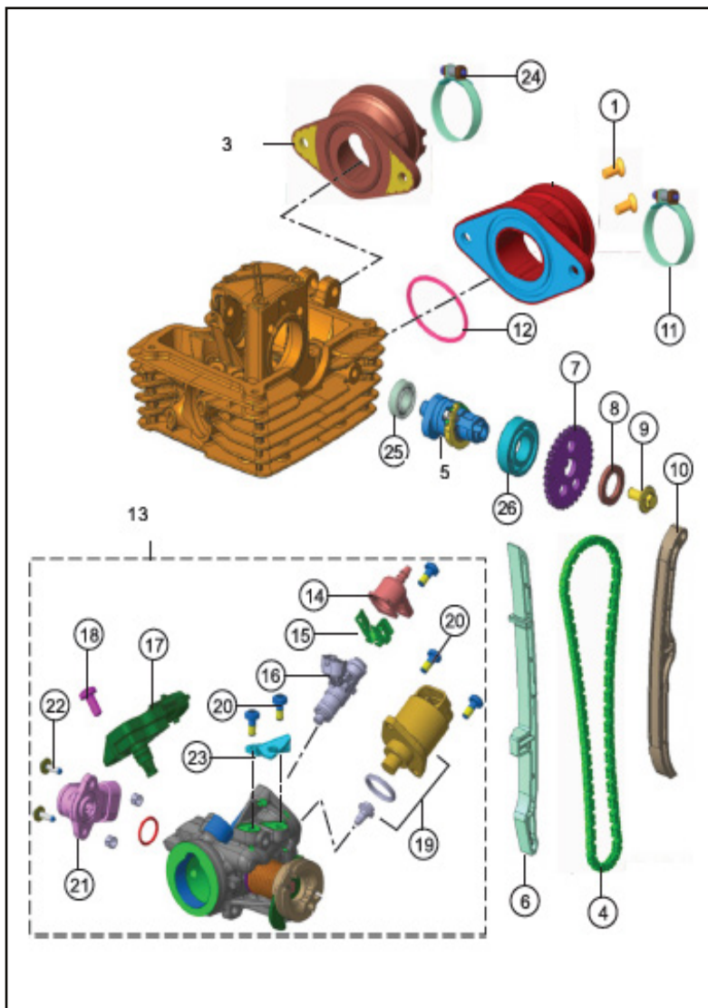
FIGURA N° 2: EJE DE LEVAS Y CUERPO DE INYECCIÓN
