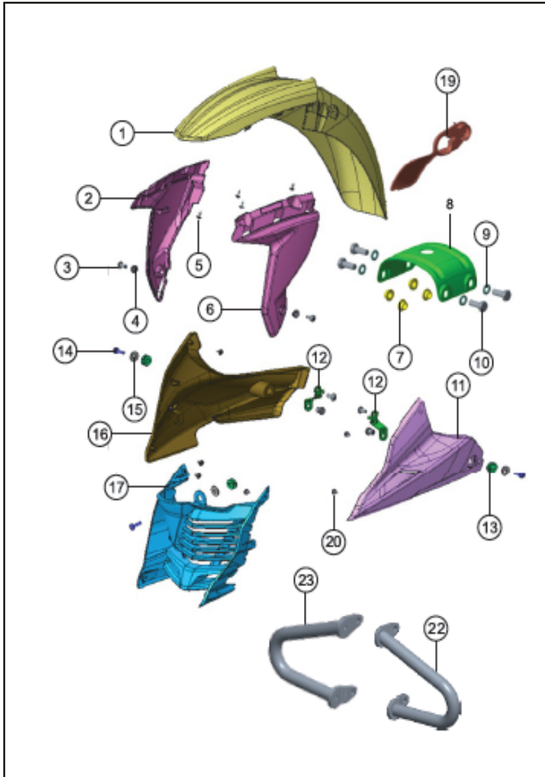
FIGURA N° 30: GUARDABARRO DELANTERO
