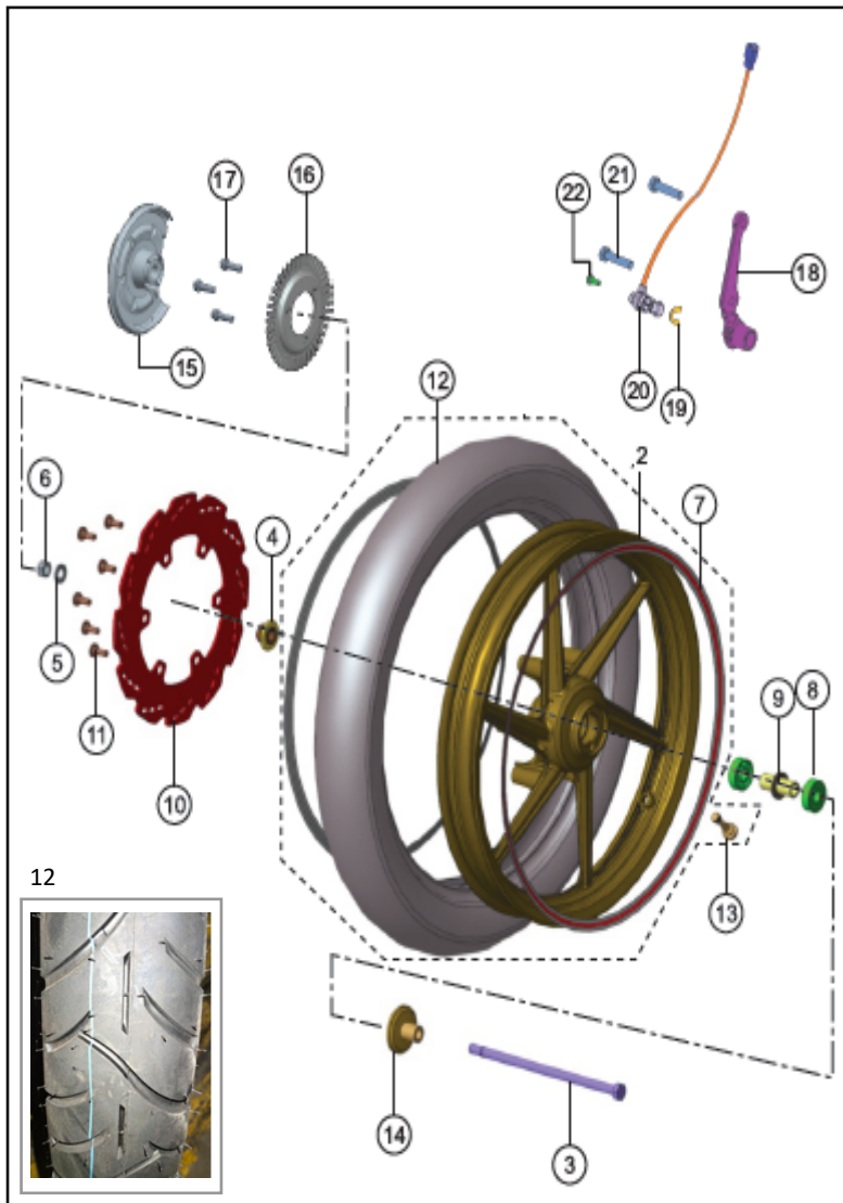
FIGURA N° 24: RUEDA DELANTERA
