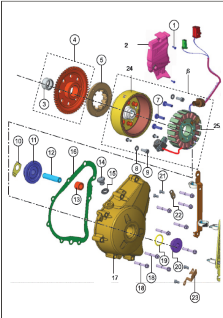
FIGURA N° 8: CUBIERTA VOLANTE / VOLANTE
