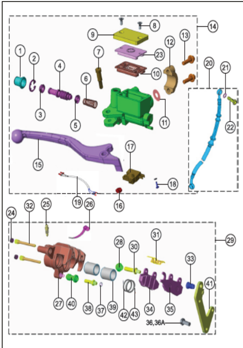
FIGURA N° 37: BOMBA FRENO DELANTERA (1/2)
