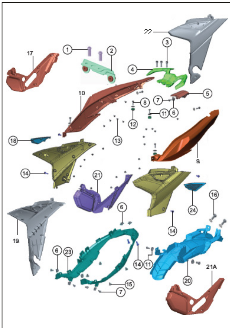
FIGURA N° 29: CUBIERTAS
