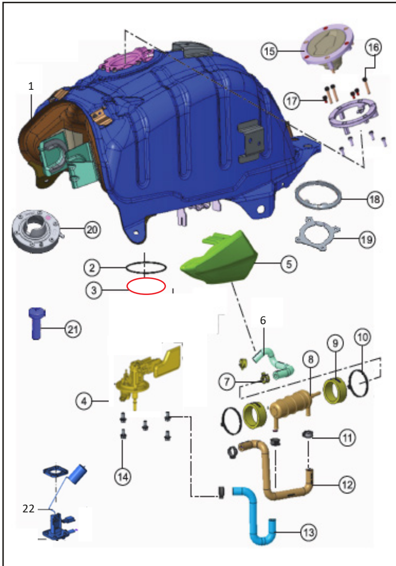
FIGURA N° 15: TANQUE DE GASOLINA Y COMPONENTES
