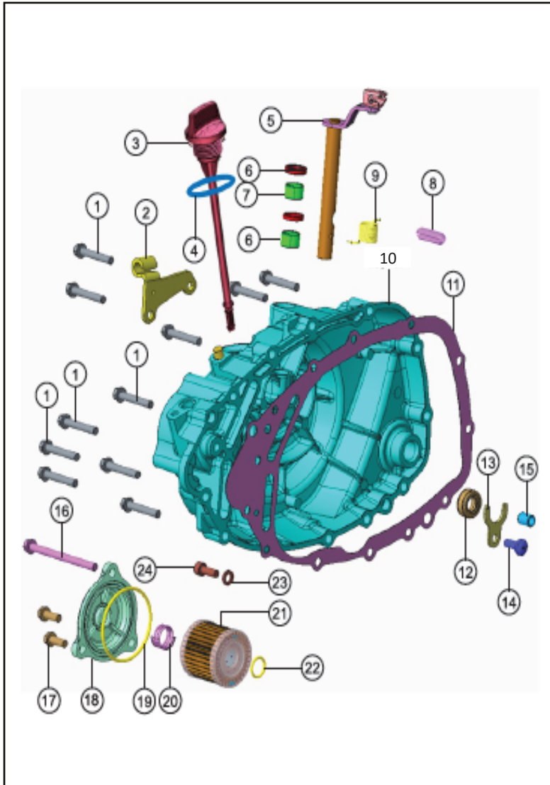
FIGURA N° 6: CUBIERTA CLUTCH
