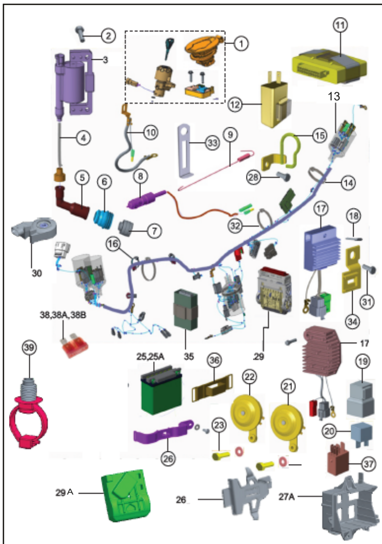
FIGURA N° 35: INSTALACIÓN ELÉCTRICA (1/2)
