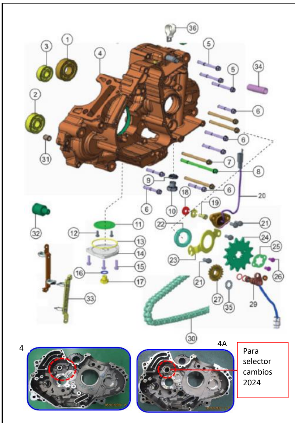
FIGURA N°5: CARCASA IZQUIERDA (1/2)
